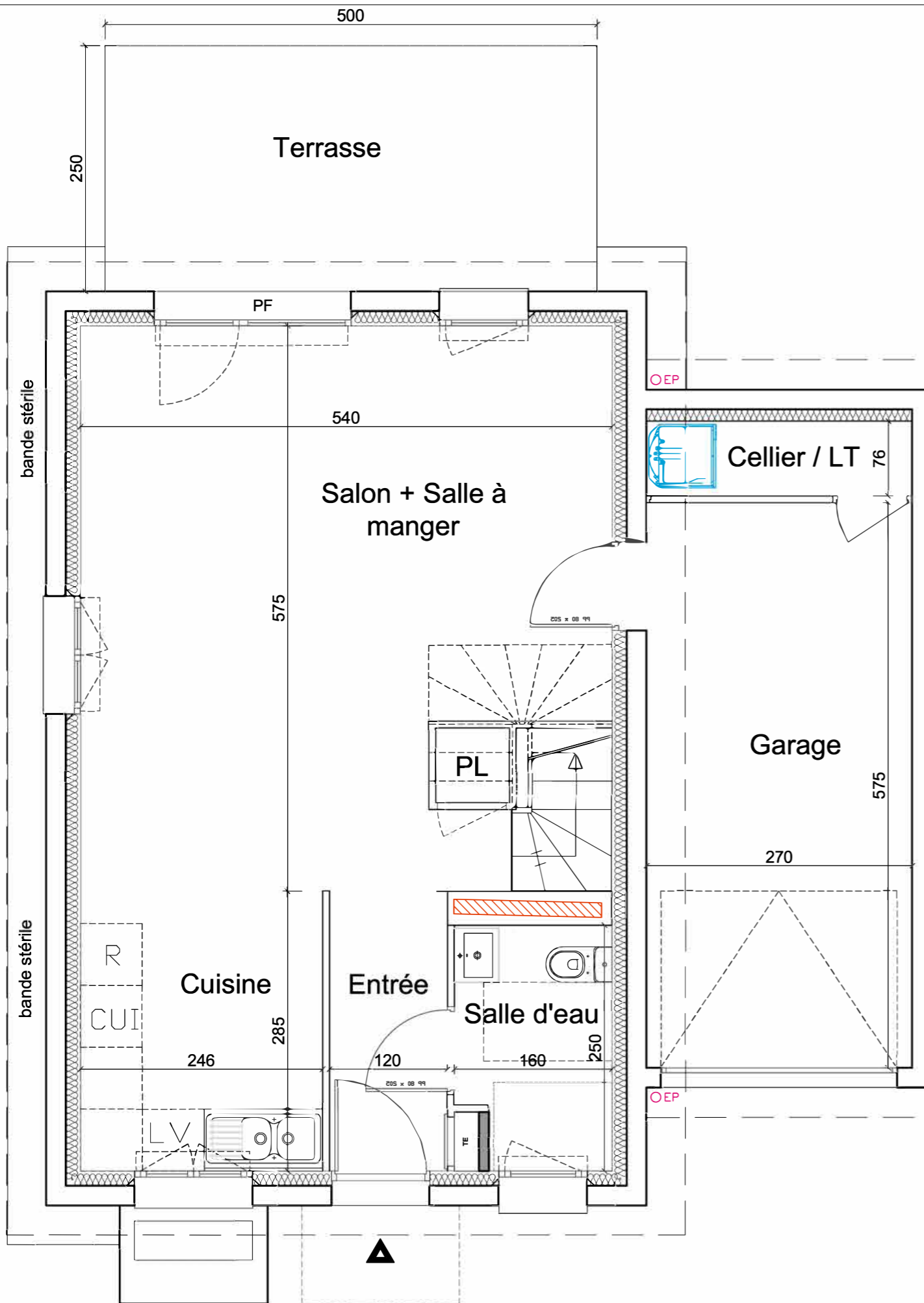
Plan niveau RdC
